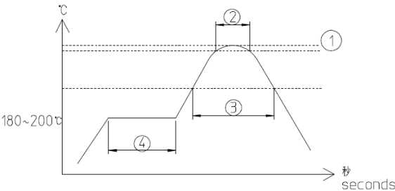
図2. リフロープロファイル Fig2. Reflow Profile
