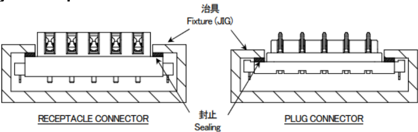
図3. 防水試験治具 Fig 3. Waterproof Test Fixture
