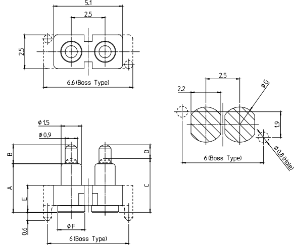
2.5mm ピッチ
