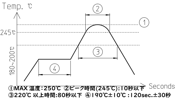
付図 2. リフロープロファイル
