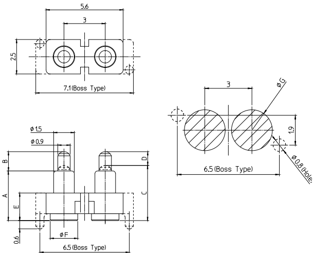
3.0mm ピッチ
