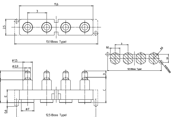
3.0mm ピッチ
