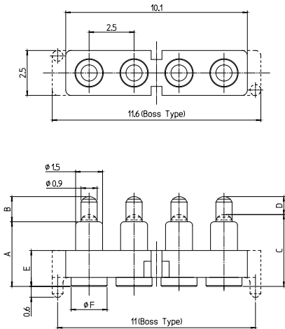
2.5mm ピッチ
