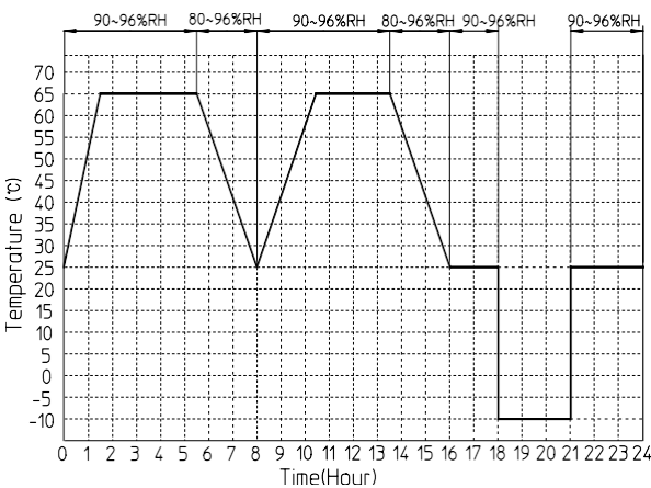
図1. 温湿度Shock Test/サイクル Fig 1. Temperature And Humidity Cycle
